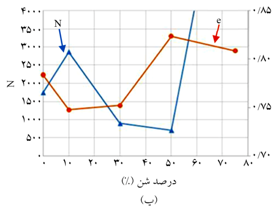
شکل (۱۴): تغییرات تعداد سیکل منجر به روانگرایی (N)، نسبت تخلخل بین ذرات ریزدانه و نسبت تخلخل دانه‌ای با درصد شن در CSR=0/1 برای نمونه‌های با تراکم نسبی مخلوط: (الف) ۱۰ درصد، (ب) ۳۰ درصد و (پ) ۵۰ درصد.
