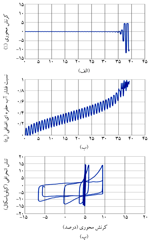
شکل (۹): نمونه نتایج آزمایش انجام شده بر روی نمونه حاوی ۳۰ درصد شن با دانسیته نسبی مخلوط برابر ۳۰ درصد در نسبت تنش تناوبی (CSR) برابر ۰/۱۵: (الف) تغییرات نسبت فشار آب حفره‌ای اضافی با تعداد سیکل‌های بارگذاری، (ب) تغییرات کرنش محوری با تعداد سیکل‌های بارگذاری، (پ) حلقه‌های تنش انحرافی-کرنش محوری.
