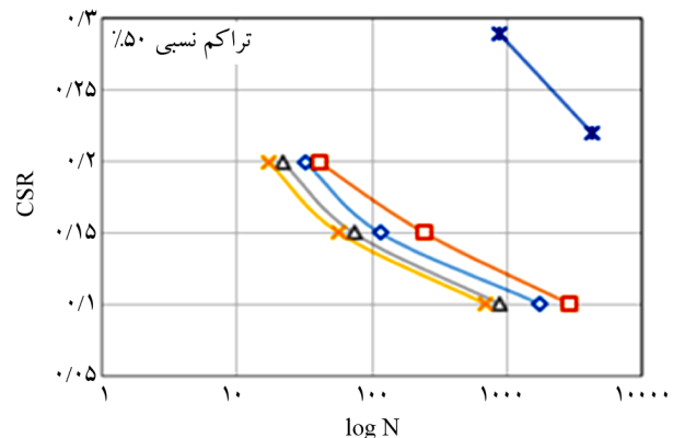
شکل (۱۱): نسبت تنش تناوبی (CSR) در برابر تعداد سیکل منجر به روانگرایی اولیه (N) برای مقادیر مختلف تراکم نسبی مخلوط.
