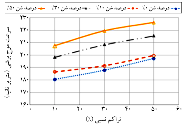
شکل (۷): تغییرات سرعت موج برشی در خاک ماسه‌ای مخلوط با شن بر حسب تراکم نسبی مخلوط و درصد شن.
