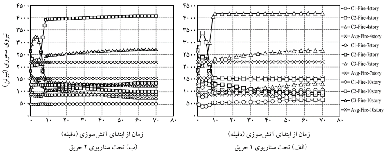
شکل (۱۱): مقایسه‌ی نیروی محوری در ستون‌های طبقه‌ی همکف قاب‌های مورد مطالعه در هر دو سناریوی حریق
