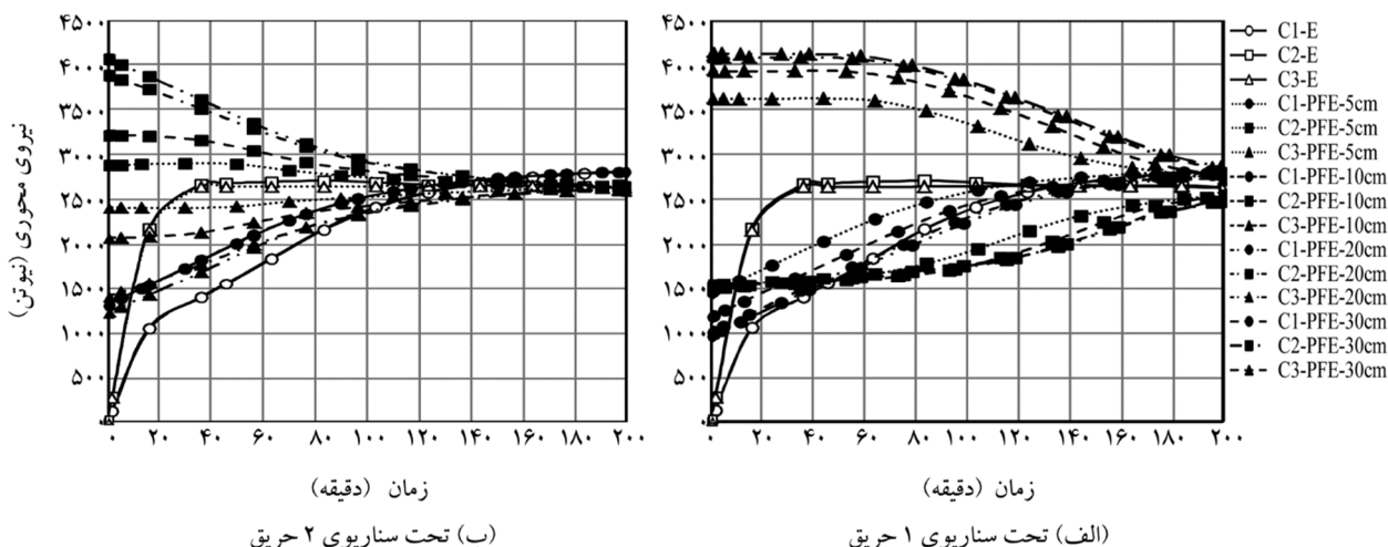
شکل (۱۲): نمودار نیروی محوری در ستون‌های طبقه‌ی همکف به هنگام زلزله قبل و پس از آتش‌سوزی برای سناریوهای حریق در قاب ۱۰ طبقه (منظور از E و PFE به ترتیب حالت زلزله و زلزله پس از آتش‌سوزی می‌باشد)
