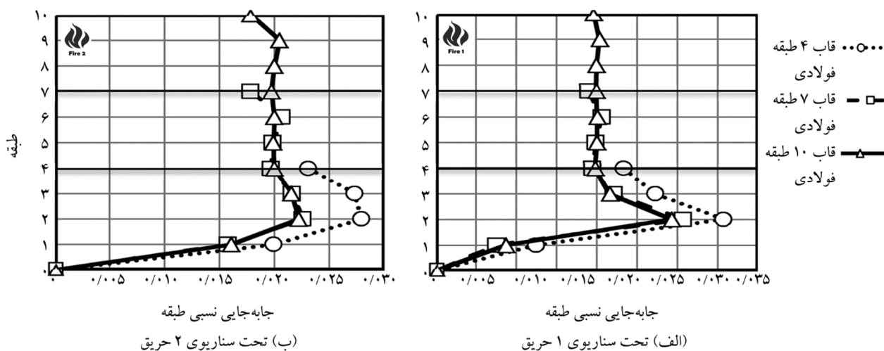
شکل (۱۵): مقایسه جابه جایی نسبی نهایی طبقات بین قاب‌های مورد مطالعه در انتهای زلزله پس از آتش سوزی
