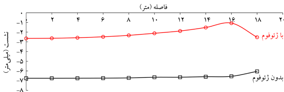
شکل (۱۲): نشست سطح زمین در حالت استاتیکی برای مدل ژئوفومی و مدل خاکی در X/a های متغیر.
