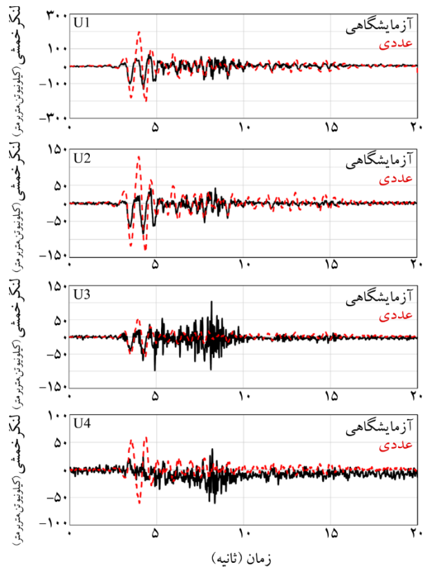
شکل (۵): مقایسه تاریخچه زمانی لنگر سقف تونل در آزمایش T2 با نتایج حاصله از مدل‌سازی عددی برای زلزله کوبه g/0.206 . PGA =
