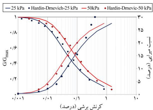
شکل (۲): منحنی G/G_{max} خاک کالیبره شده با مدل هاردین-درینویج.
