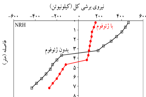
شکل (۱۸): مقایسه نیروهای برشی لرزه‌ای و کل در طول دیواره برای مدل ژئوفومی و مدل خاکی در زلزله نورث‌ریج.
