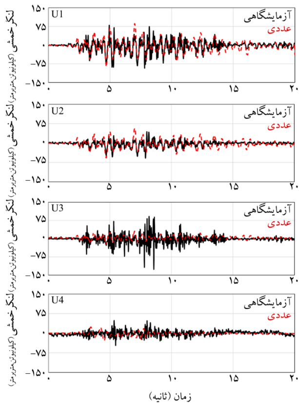
شکل (۷): مقایسه تاریخچه زمانی لنگر سقف تونل در آزمایش T2 با نتایج حاصله از مدل سازی عددی برای زلزله نورتریج g = 0.186 PGA.
