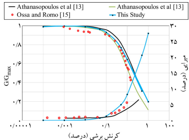
شکل (۹): چرخه هیستریزس تنش-کرنش و نمودار کاهش مدول برشی ژئوفوم برای المان وسط مدل T2 در PGA = 0.3 \text{ g} .
