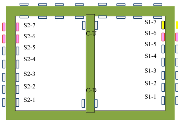
شکل (۳): ابزارگذاری سازه تونل برای برداشت لنگرهای خمشی سازه تونل.
