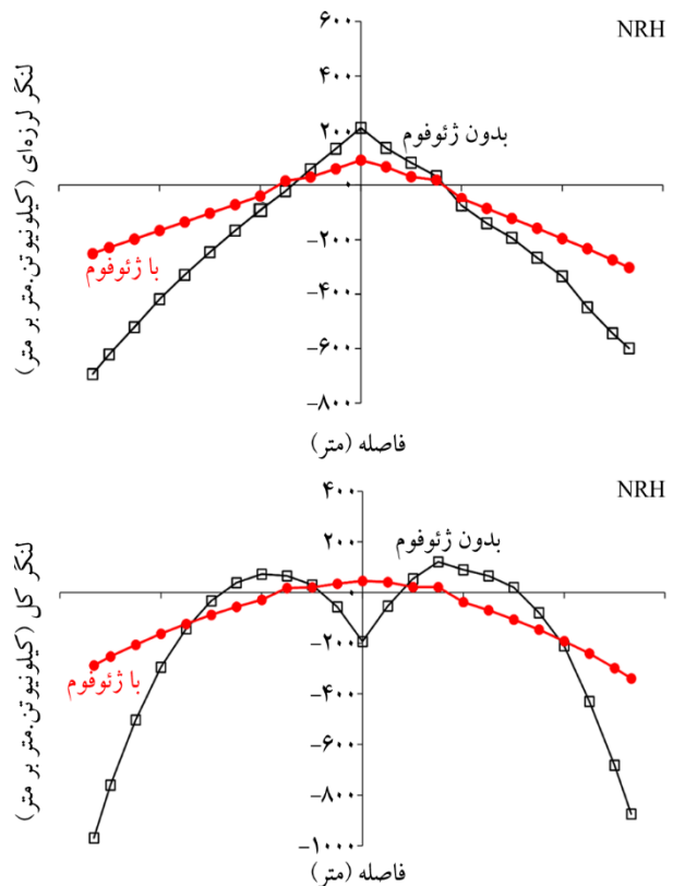
شکل (۱۹): مقایسه لنگرهای لرزه‌ای و کل در سقف برای مدل ژئوفومی و مدل خاکی در زلزله نورتریج.
