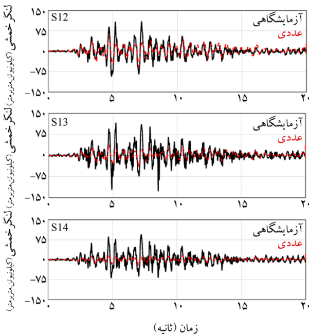
شکل (۶): مقایسه تاریخچه زمانی لنگر دیواره تونل در آزمایش T2 با نتایج حاصله از مدل‌سازی عددی برای زلزله نورث‌ریج g/0.186 . PGA =
