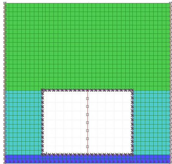
شکل (۱): شبکه‌بندی مدل آزمایشگاهی T2 در نرم‌افزار FLAC 2D.
