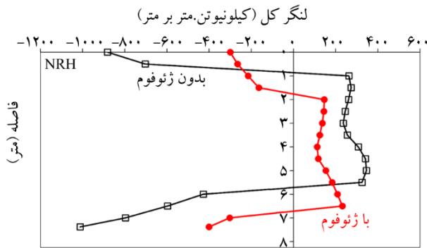
شکل (۱۷): مقایسه لنگرهای لرزه‌ای و کل در طول دیواره برای مدل ژئوفومی و مدل خاکی در زلزله نورث‌ریج.
