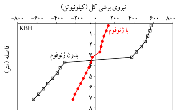
شکل (۱۴): مقایسه نیروهای برشی لرزه‌ای و کل در طول دیواره برای مدل ژئوفومی و مدل خاکی در زلزله کوبه.
