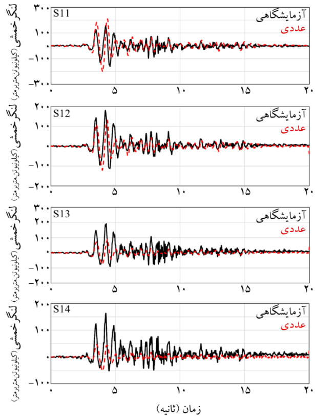
شکل (۴): مقایسه تاریخچه زمانی لنگر دیواره تونل در آزمایش T2 با نتایج حاصله از مدل‌سازی عددی برای زلزله کوبه g/0.206 . PGA =
